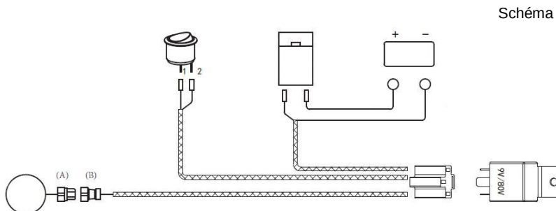
Schéma de montage
