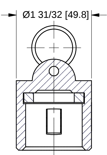
SECTION A-A SCALE 1 : 1
