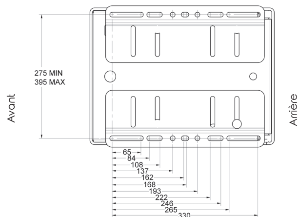
Plaque d'adaptation
